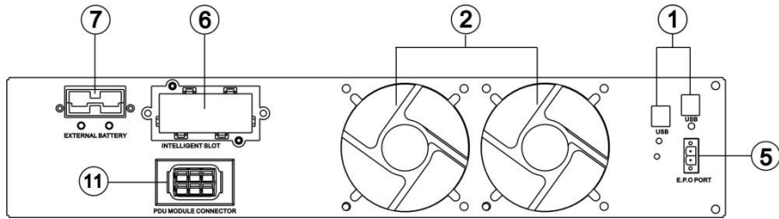
3KVA 機架臥式 UPS
