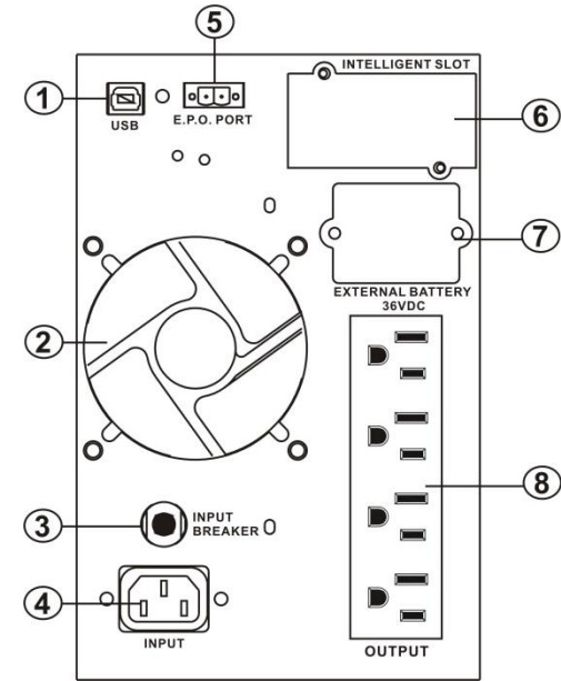
1KVA 立式 UPS
