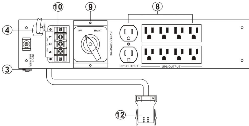
3KVA 機架臥式 UPS 之電源分配器 PDU
