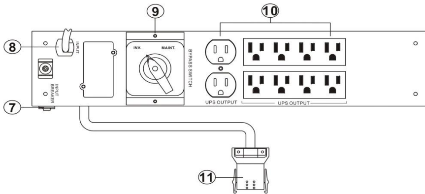
1KVA 機架臥式 UPS 之電源分配器 PDU
